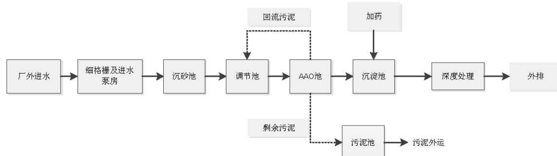
图9 污水处理厂污水处理工艺流程图
