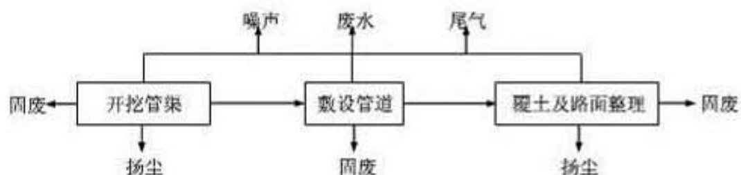
图 8 工程配套管网施工工艺流程
